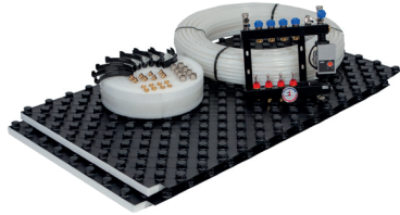
Set vloerverwarming
